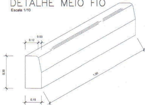
DETALHE MEIO FIO
