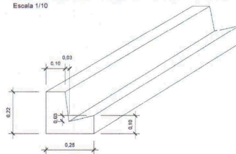
DETALHE MEIO FIO COM SARJETA
